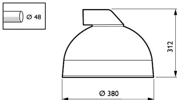
Rozměrové výkresy
