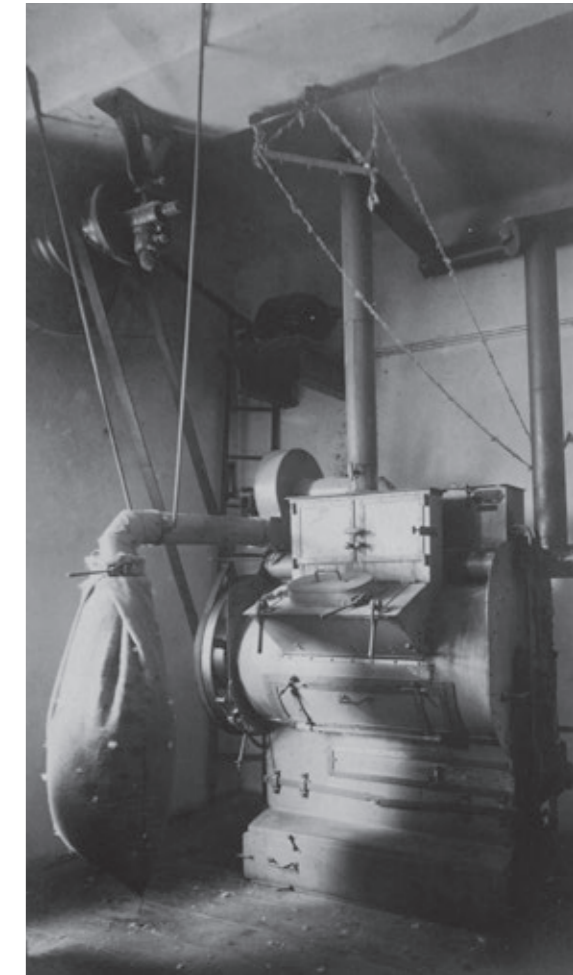
Jeden ze strojů na zpracování peří
